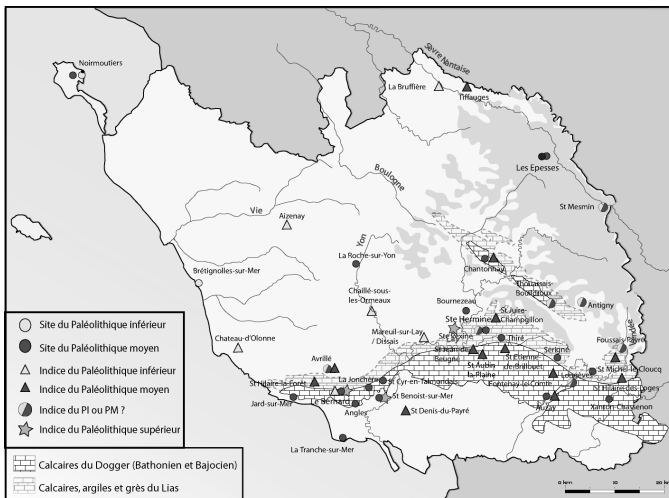
Carte de répartition des sites paléolithiques de Vendée, par rapport aux formations géologiques (réalisation S. Bourdin-Launay).
